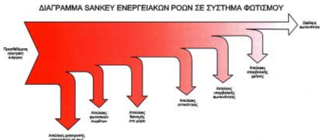
Σχήμα 4.19. Ενεργειακές ροές σε εγκατάσταση τεχνητού φωτισμού
