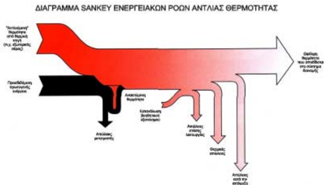
Σχήμα 4.16. Ενεργειακές ροές σε συγκρότημα κεντρικής αντλίας θερμότητας (λειτουργία θέρμανσης)
