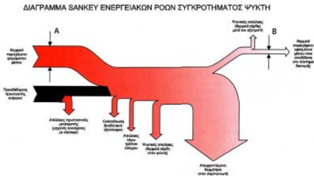
Σχήμα 4.15. Ενεργειακές ροές σε συγκρότημα κεντρικού ψύκτη κλιματισμού
