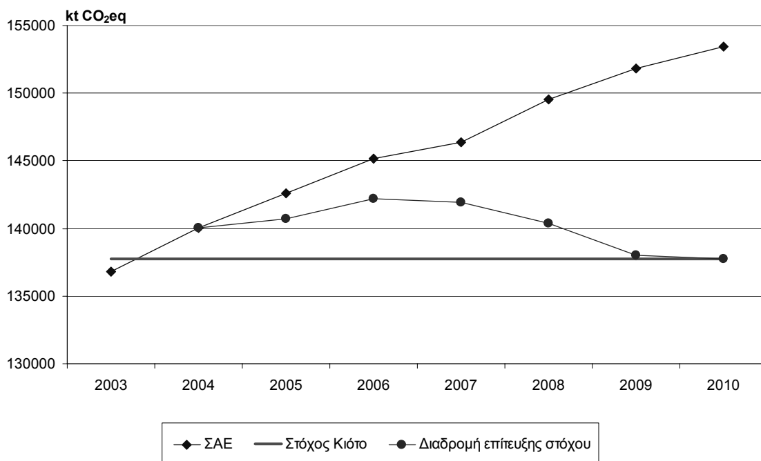
Σχήμα 1-1: ΣΑΕ και επιλεγείσα διαδρομή για την επίτευξη του στόχου του Κιότο για τη Ελλάδα το 2010.
