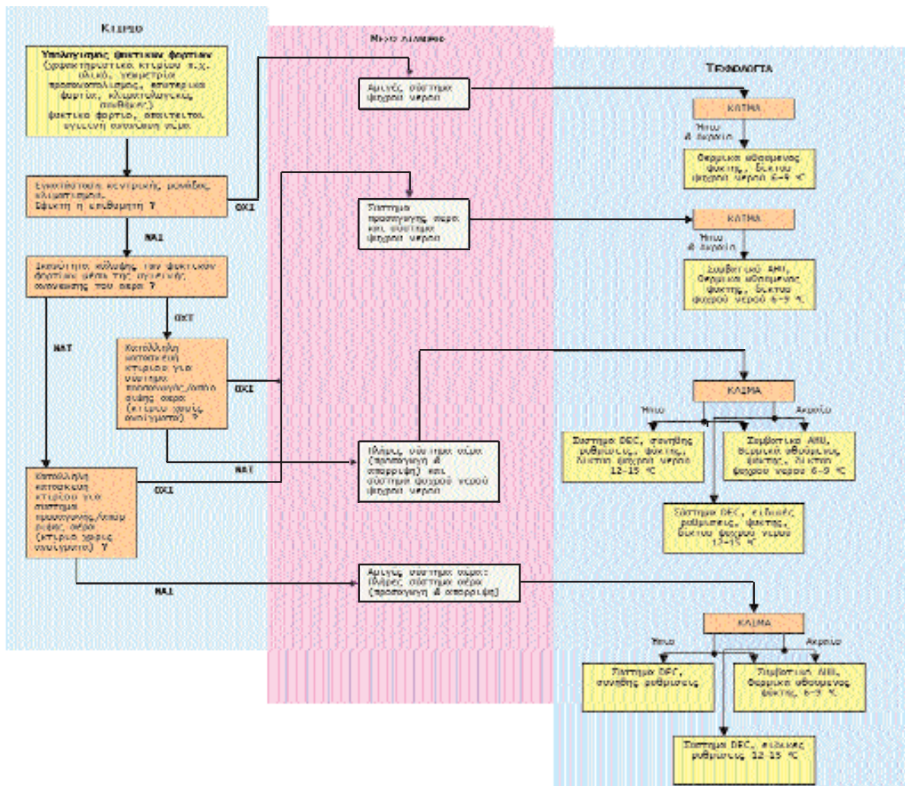
Σχίμα 10 Διάγραμμα διαδικασίας λήψης απόφασης για τεχνολογίες ηλιακού κλιματισμού Συνομογραφία: DEC Desiccant cooling, AHU Air Handling Unit
