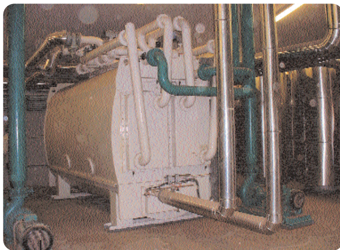
Φωτογραφία 6 Ψύκτης προσρόφησης 350kW - Βιομηχανία Σαράντης Α.Ε.- Ελλάδα
