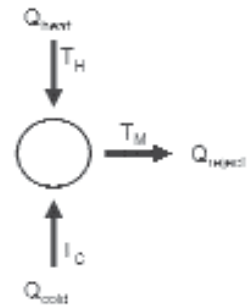
Σχήμα 6 Βασικό σχήδιο της διαδικασίας: Το Q_{cold} είναι η θερμότητα που απορρίπτεται από το ψυχρό νερό στον εξατμιστή του ψύκτη (ψυκτική ενέργεια), το Q_{heat} είναι η απαιτούμενη θερμότητα αναγέννηση (τροφοδοσίας), και το ποσό Q_{reject} , το άθροισμα του Q_{cold} και του Q_{heat} , πρέπει να απορριφθεί σε μέσο επίπεδο θερμοκρασίας T_m . Το Q_{heat} παρέχεται είτε από το ηλιακό σύστημα είτε από τις εφεδρικές πηγές θερμότητας, π.χ. από τηλεθέρμανση ή από καυστήρα φυσικού αερίου.
