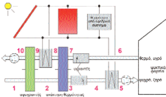
Σχήμα 9 Σχηματικό διάγραμμα ενός συστήματος ψύξης DEC
