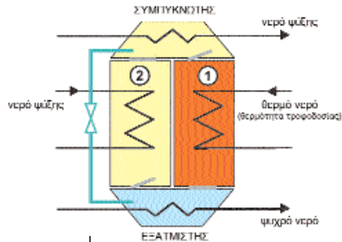
Σχήμα 8 Σχηματικό διάγραμμα ενός ψύκτη προσρόφησης
