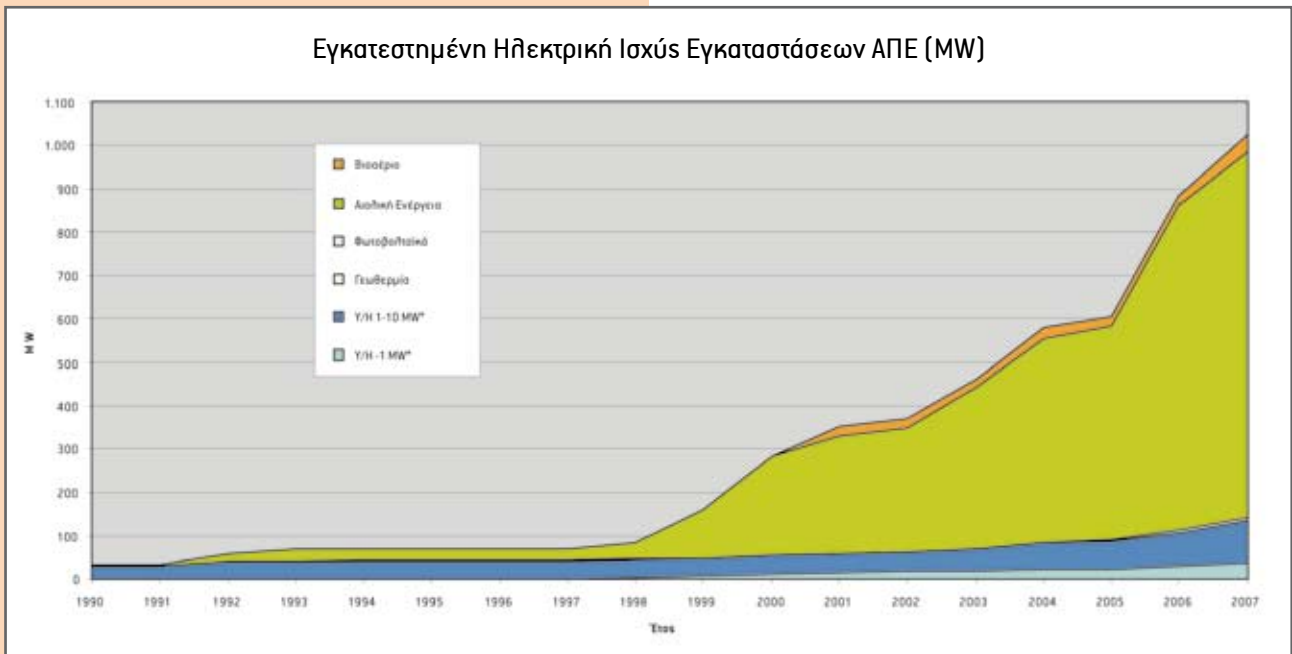
Διάγραμμα 1: Εξέλιξη εγκατεστημένης ισχύος ΑΠΕ χωρίς μεγάλα υδροηλεκτρικά
