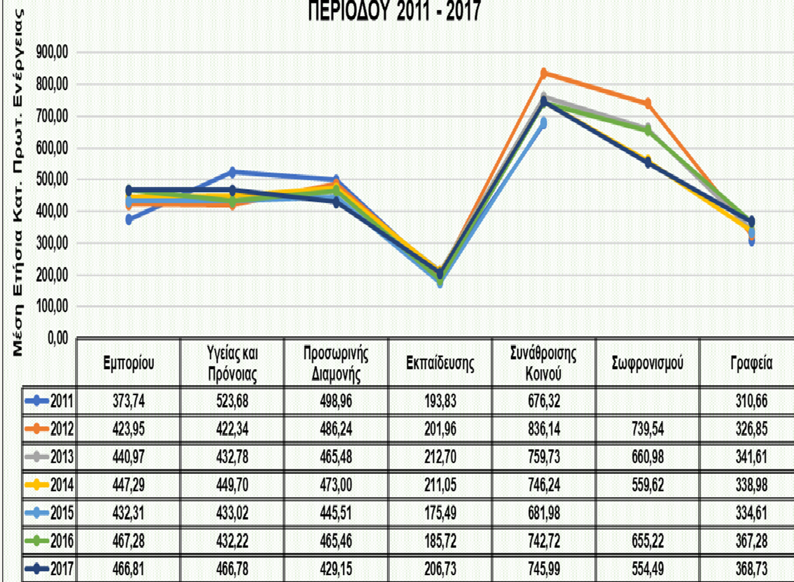
ΜΕΣΗ ΕΤΗΣΙΑ ΕΝΕΡΓΕΙΑΚΗ ΚΑΤΑΝΑΛΩΣΗ ΚΤΙΡΙΩΝ ΤΡΙΤΟΓΕΝΟΥΣ ΤΟΜΕΑ ΠΕΡΙΟΔΟΥ 2011 - 2017
