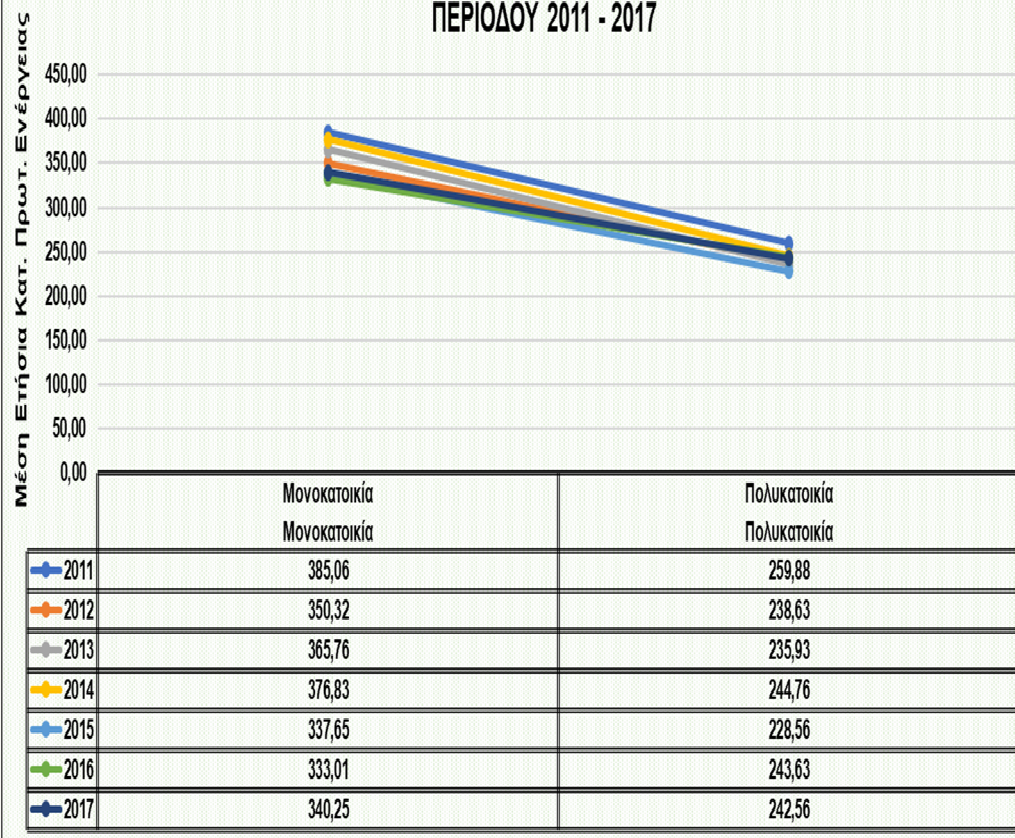
ΜΕΣΗ ΕΤΗΣΙΑ ΕΝΕΡΓΕΙΑΚΗ ΚΑΤΑΝΑΛΩΣΗ ΚΤΙΡΙΩΝ ΚΑΤΟΙΚΙΑΣ ΠΕΡΙΟΔΟΥ 2011 - 2017
