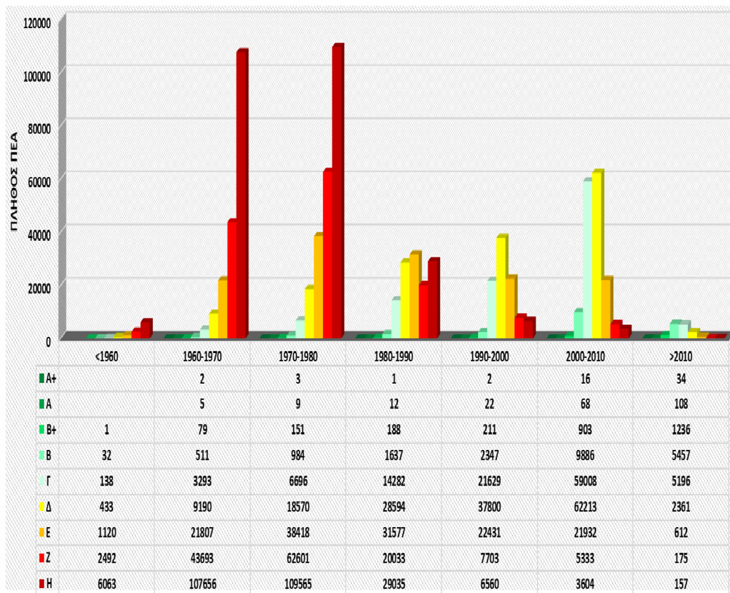
ΠΛΗΘΟΣ ΠΕΑ ΚΤΙΡΙΩΝ ΚΑΤΟΙΚΙΑΣ ΑΝΑ ΔΕΚΑΕΤΙΑ ΚΑΤΑΣΚΕΥΗΣ ΚΑΙ ΕΝΕΡΓΕΙΑΚΗ ΚΑΤΗΓΟΡΙΑ
