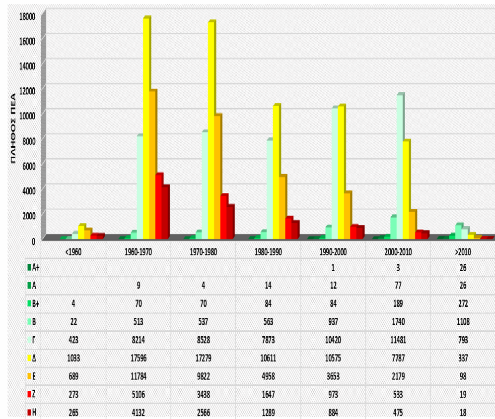
ΠΛΗΘΟΣ ΠΕΑ ΚΤΙΡΙΩΝ ΤΡΙΤΟΓΕΝΟΥΣ ΤΟΜΕΑ ΑΝΑ ΔΕΚΑΕΤΙΑ ΚΑΤΑΣΚΕΥΗΣ ΚΑΙ ΕΝΕΡΓΕΙΑΚΗ ΚΑΤΗΓΟΡΙΑ
