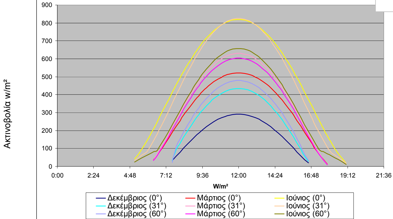
Όλική Ημερήσια Οριζόντια Ακτινοβολία (Αθήνα)
