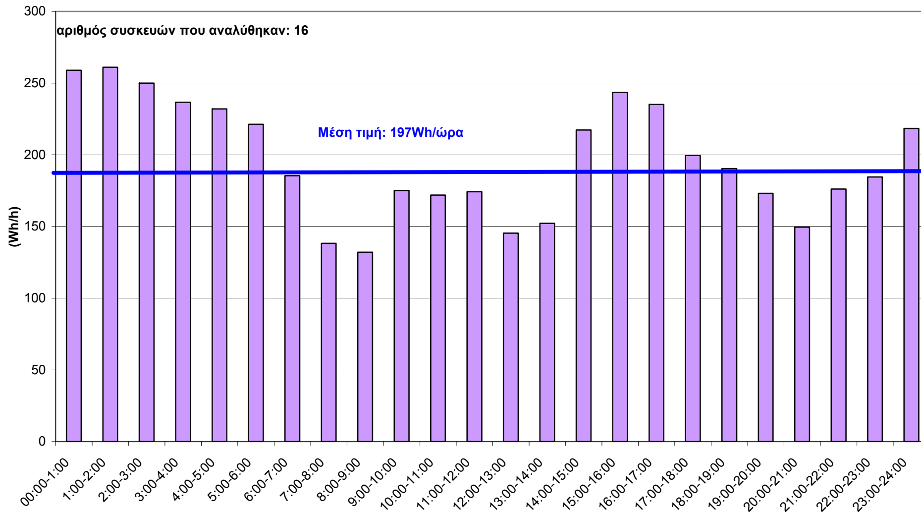
Ημερήσια Καμπύλη Φορτίου (Wh/ώρα)
